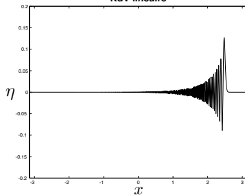
KdV linéaire
