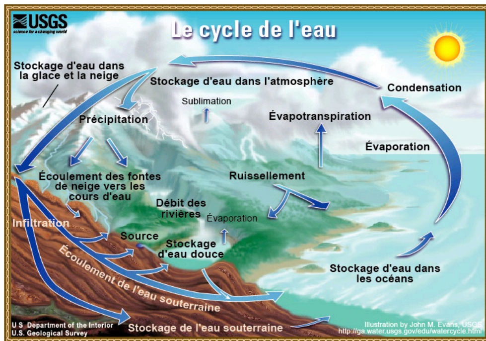
FIG. 1 – Le cycle de l'eau. Schéma USGS.
