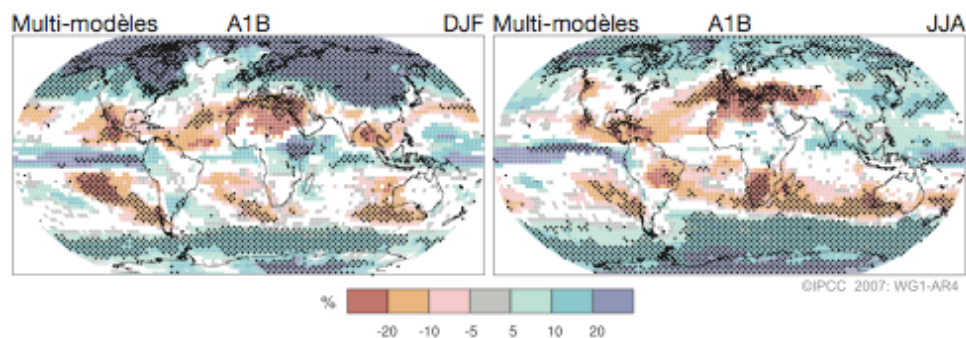
FIG. 4 – Simulation de la répartition des modifications des précipitations d'ici la fin du XXI e siècle. a) Hiver. b) Été. Rapport IPCC 2007.
