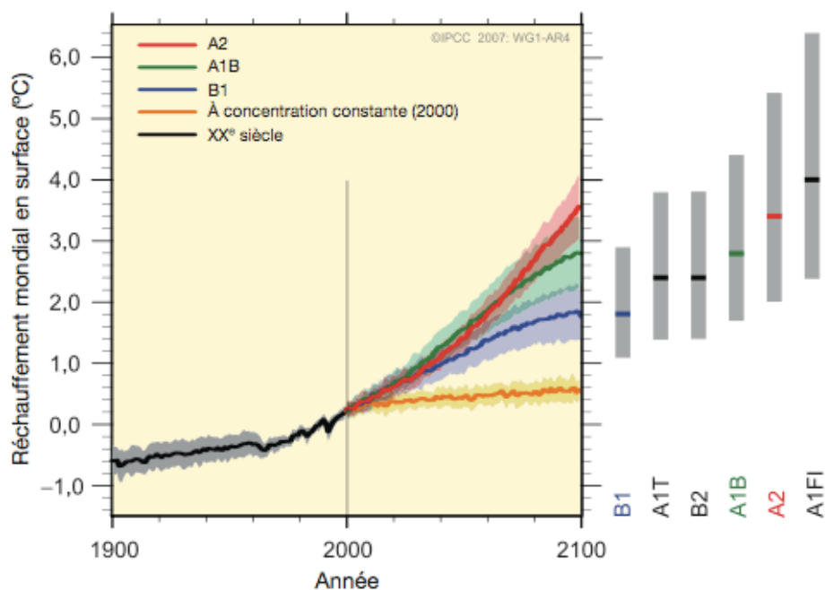
FIG. 3 – Moyennes des multi-modèles et fourchettes estimées du réchauffement en surface. Rapport IPCC 2007.
