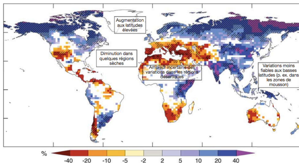
FIG. 5 – Projections et cohérence des simulations concernant les variations relatives du ruissellement d'ici la fin du XXI e siècle. Rapport IPCC 2007.
