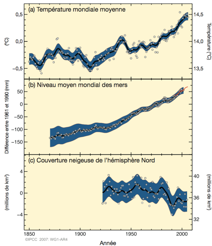
FIG. 2 – Changements de température, du niveau des mers et de la couverture neigeuse dans l'hémisphère Nord. Rapport IPCC 2007.
