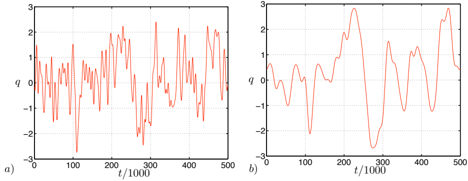
Figure 4.9: Condition aux limites amont aléatoire q(t) pour q_m = 1 . a) \sigma_q = 3 \cdot 10^3 . b) \sigma_q = 9 \cdot 10^3 .
